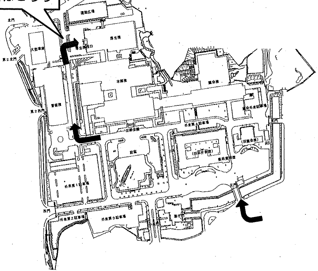
県庁舎内全体配置図
